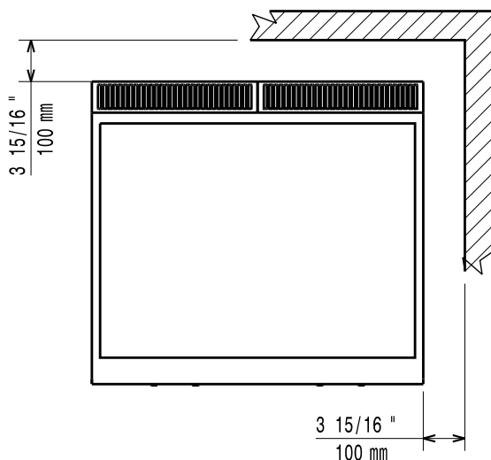
Planta
